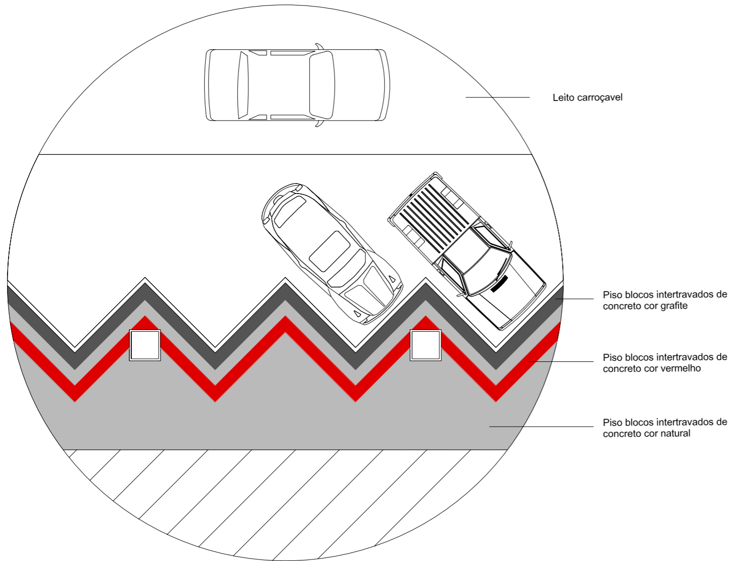
DETALHE PAGINAÇÃO ESC.: 1/100
